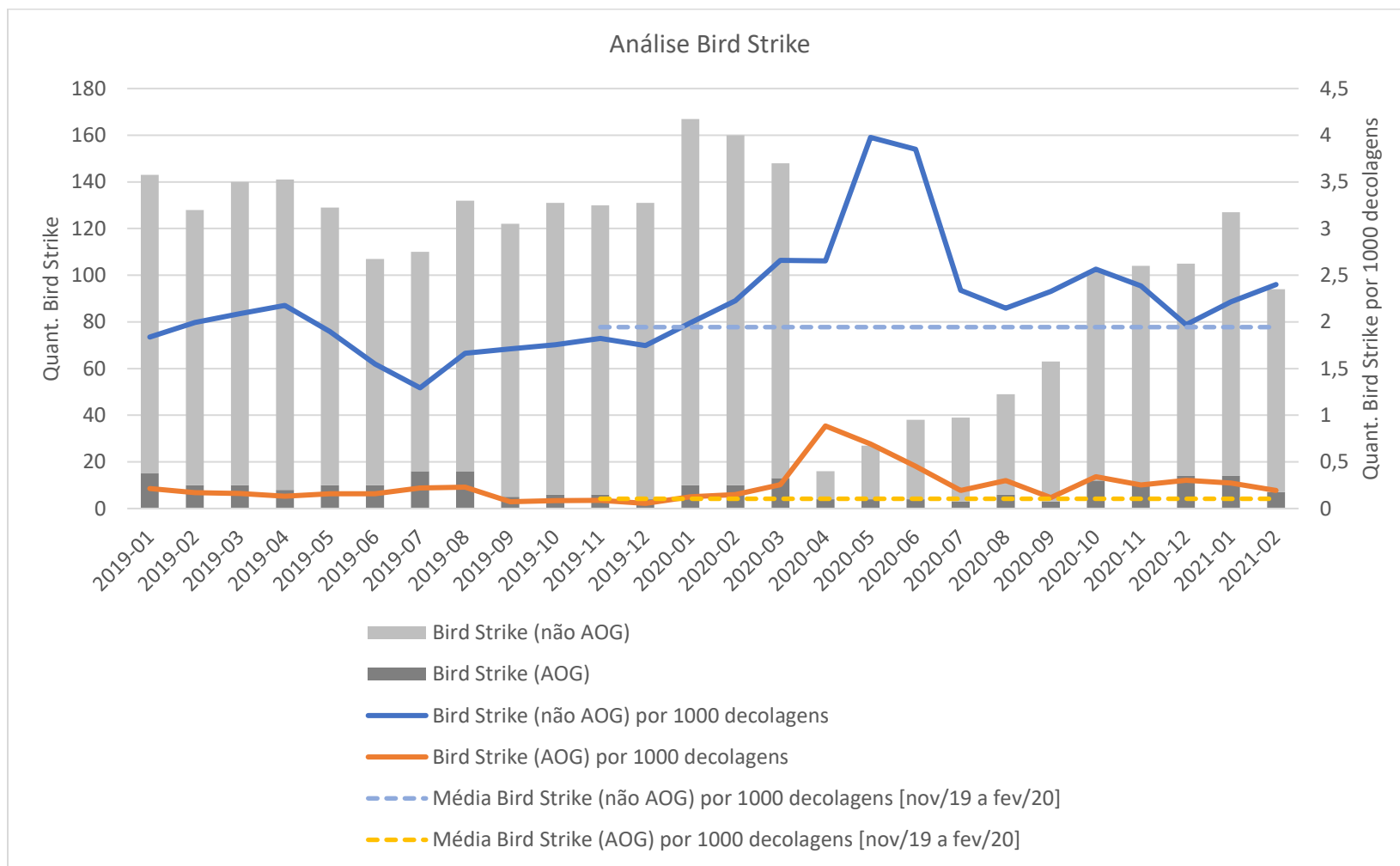
Figura 1- Análise de Bird Strike realizada pelo grupo de trabalho BCAST COVID-19
